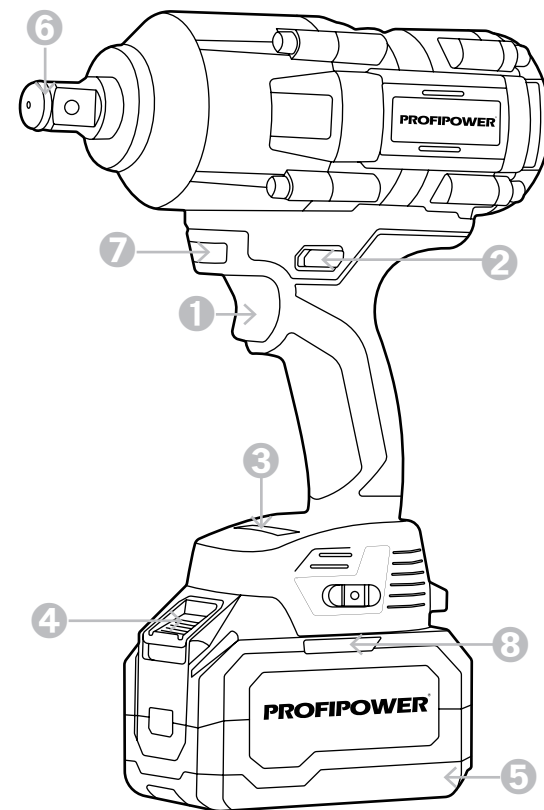
Рисунок 1.4.1. Устройство инструмента
